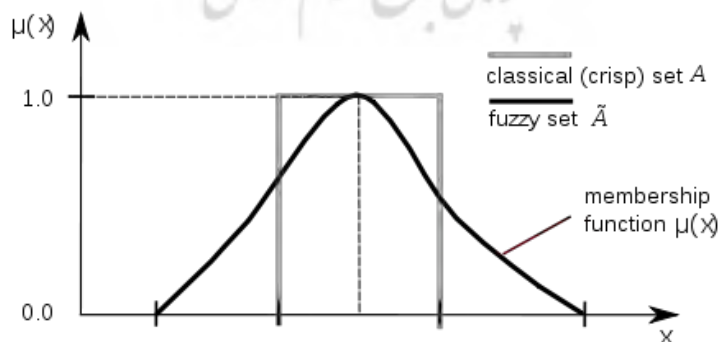
شکل شماره ۴: تابع عضویت یک مجموعه فازی
