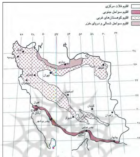
شکل شماره ۱- تقسیم بندی چهارگانه‌ی حوزه‌های جغرافیایی و اقلیمی ایران
