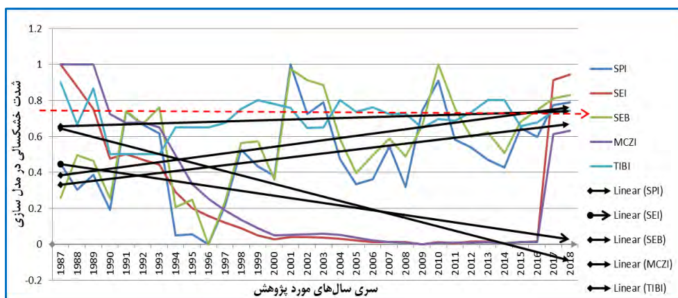
شکل ۶. نمودار نوسان شاخص‌ها در ایستگاه اسلام‌آباد غرب در مقیاس ۶ ماهه در دوره آماری (۱۹۸۷-۲۰۱۸)
