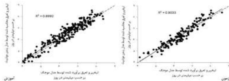
شکل ۸- نمودار پراکنش تبخیر و تعرق محاسبه شده توسط مدل پنمن موتیت و برآورد شده توسط مدل موجک تحت سناریوی سوم
