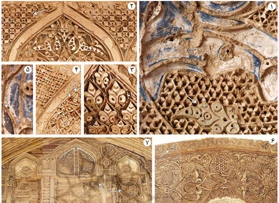
تصویر ۱۲. عکس ۱) بخشی از رنگ آمیزی محراب مسجد جامع فریومد: رنگ سفید برای زیرسازی رنگ آبی لاجوردی در زمینه گچبری و رنگ سبز برای طرح برگ مانند؛ ۲) بخشی از مقرنس گچی ایوان جنوبی مسجد جامع فریومد که با رنگ های قرمز، مشکی و سفید رنگ آمیزی شده است؛ ۳) بخش دیگری از مقرنس ایوان جنوبی مسجد جامع فریومد با رنگ آمیزی سفید، سیاه و قرمز؛ ۴) بخشی از مقرنس ایوان جنوبی مسجد جامع فریومد به رنگ های سفید و قرمز؛ ۵) بخشی از رنگ آمیزی محراب مسجد جامع فریومد با رنگ های سفید، آبی و سیاه؛ ۶) بخشی از زیر طاق ایوان شمال غربی رباط شرف حاوی رنگ های زرد، سفید و سیاه؛ ۷) ایوان ورودی حیاط دوم رباط شرف، پیکان های سفید رنگ زرد را مشخص می کنند؛ ماخذ: نگارنده.
