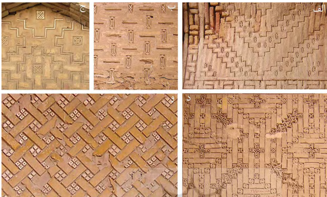
تصویر ۲. الف- شیوه شبه آجری ساده در زیر طاق رباط شرف؛ ب) شیوه شبه آجری در دیواره‌ها؛ ج) طرح گل انداز آجری به شیوه شبه آجری در طاق‌ما؛ د) طرح گل انداز آجری پُرکار با نقوش گیاهی در کلوک‌بندها؛ و) طرحی غیر معمول در شیوه شبه آجری (حصیر بافت)، مأخذ: نگارنده.
