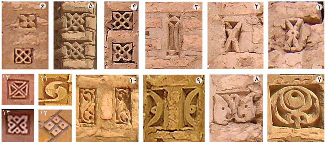
تصویر ۳. کلوک‌بندهای گچی رباط شرف، ماخذ: نگارنده؛ نقوش ۱-۳ از انواع نقوش ساده و پُرکار بر در رباط شرف هستند؛ نقوش ۴-۶ و ۱۲-۱۴ از انواع نقوش هندسی بر زمینه مربع هستند؛ شماره‌های ۷، ۸، ۹ و ۱۰ سه نوع نقش گیاهی و شماره ۱۱ نقشی اسلیمی است؛ شماره‌های ۹ و ۱۰ دو نقش را در بین بند آجر عمودی نشان می‌دهد که جفت هستند.
