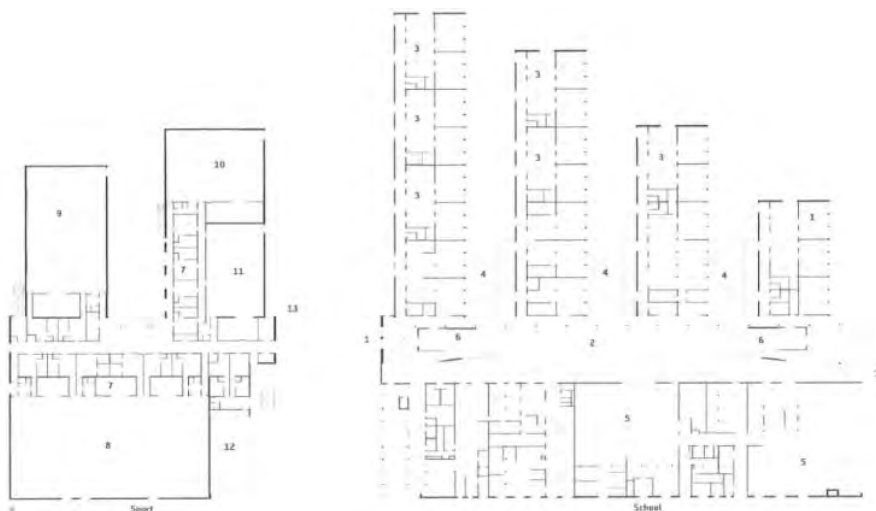
تصویر ۱۱. مدرسه تریاس وی ام بی، بهره‌گیری از الگوی ۲ در چیدمان کلاس‌ها و الگوی ۱ در چیدمان فضای خدماتی و الگوی ۱ در چیدمان فضای عطف اصلی (همان، ۲۱۰)
