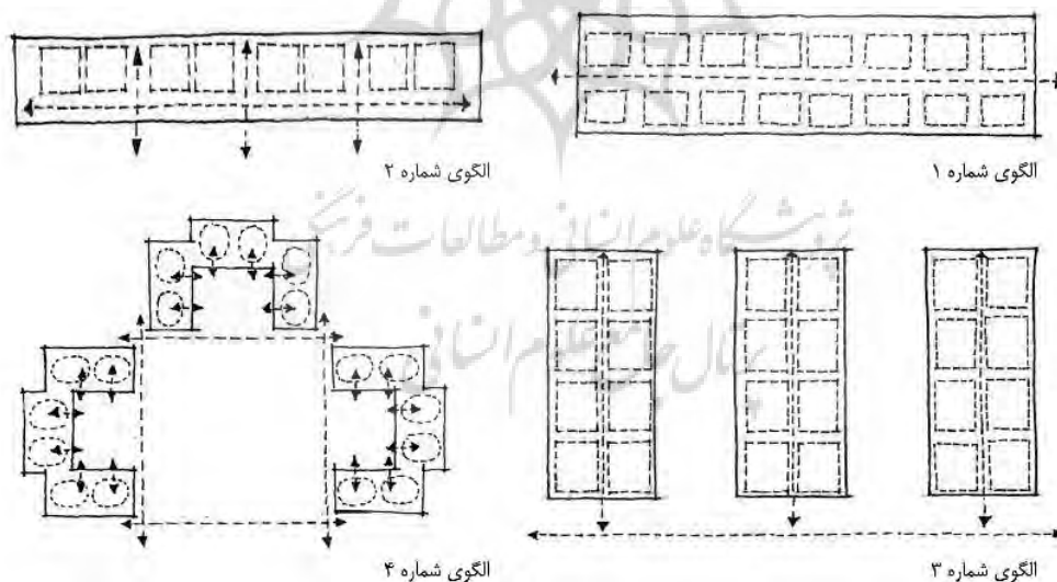
تصویر ۱. معرفی مصور الگوهای مختلف چیدمان کلاس‌ها در بناهای آموزشی (همان، ۹۲-۹۸)
