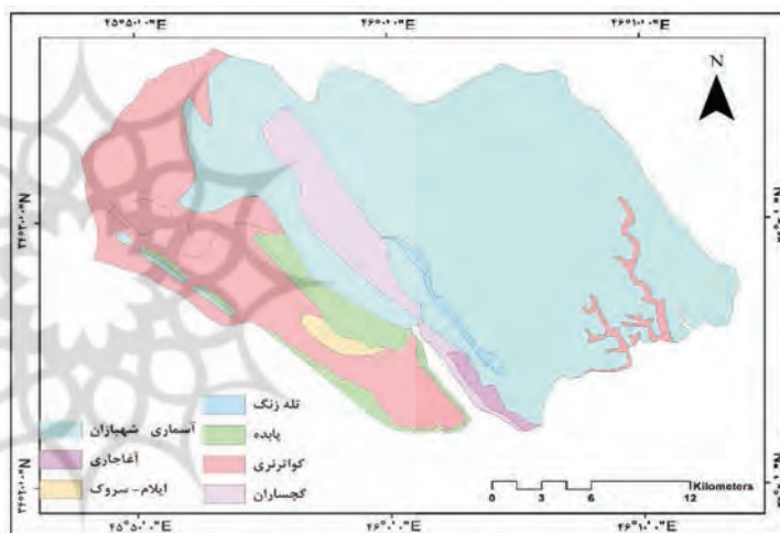
نگاره ۲: نقشه زمین‌شناسی توده‌های آهکی دالاهو
