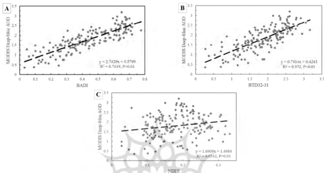
شکل ۷: تحلیل رگرسیون بین MODIS Deep Blue AOD و BADI (A) و BTD ۳۲-۳۱ (B) و NDDI (C) برای موج طوفان گردوغبار ۱۷ ژوئیه ۲۰۱۶.
