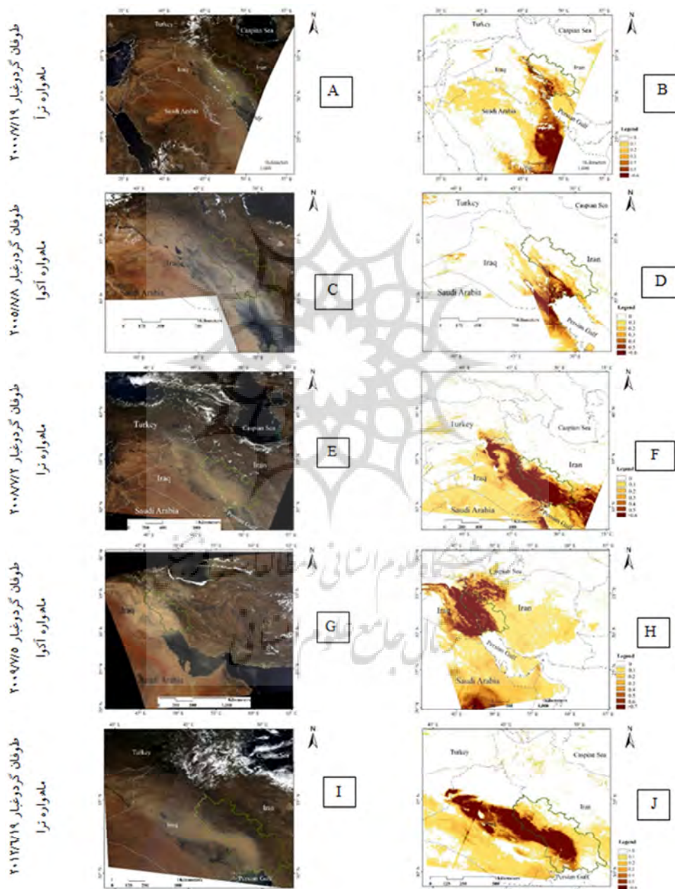
شکل ۵: استفاده از شاخص BADI برای ۵ موج طوفان گردوغبار. A, C, E, G و I به ترتیب تصاویر رنگی حقیقی موج طوفان‌های گردوغبار ۱۹ ژوئیه ۲۰۰۰، ۸ اوت ۲۰۰۵، ۲ ژوئیه ۲۰۰۸، ۵ ژوئیه ۲۰۰۹، ۱۹ ژوئن ۲۰۱۲ می‌باشد. B, D, F, H و J به ترتیب نقشه پهنه‌بندی شاخص BADI موج طوفان‌های گردوغبار ۱۹ ژوئیه ۲۰۰۰، ۸ اوت ۲۰۰۵، ۲ ژوئیه ۲۰۰۸، ۵ ژوئیه ۲۰۰۹، ۱۹ ژوئن ۲۰۱۲ می‌باشد.
