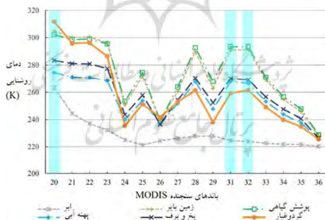
شکل ۲: ویژگی‌های دمای روشنایی اسپکترورادیومتر تصویربردار با قدرت تفکیک متوسط ۲
