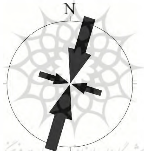
شکل ۱۱. موقعیت تنش‌های اصلی بیشینه (۰۱۷/۰۲) و میانه (۱۰۷/۰۰) به دست آمده از کل داده‌های گسلی در منطقه مورد مطالعه پس از چرخش داده‌ها. (محور تنش اصلی کمینه قائم است.)
