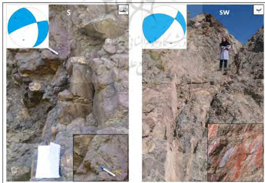
شکل ۵. تصویر صحرایی از گسل‌های برداشت شده در عملیات صحرایی، الف) گسل F15 از نوع معکوس با مولفه‌ی امتداد لغز چپگرد، ب) گسل F13 از نوع معکوس با مولفه‌ی امتداد لغز چپگرد.
