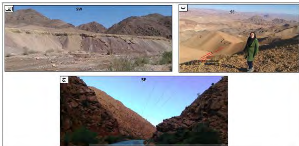
شکل ۱۳. پدیده‌های ریخت‌زمین ساختی منطقه‌ی مورد مطالعه، الف) تراس آبرفتی مربوط به حوضه‌ی شماره‌ی ۳۳، ب) انحراف آبراهه توسط گسل امتدادلغز چپگرد در حوضه‌ی شماره‌ی ۴۴، ج) دره‌ی V شکل مربوط به حوضه‌ی شماره‌ی ۲۴.
