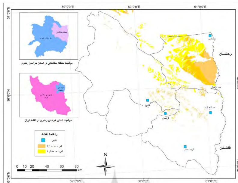
شکل ۵: نقشه پراکندگی رسوبات لسی بر مبنای نقشه های زمین شناسی ۱:۲۵۰۰۰۰ و ۱:۱۰۰۰۰۰.
