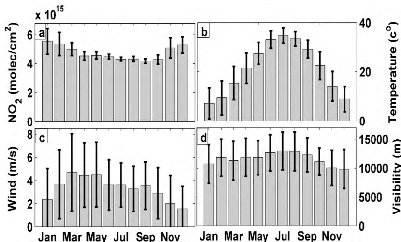
شکل (۵). میانگین ماهانه مشترک (a) دی اکسید نیتروژن، (b) دمای سطحی، (c) باد و (d) دید افقی شهر مشهد
