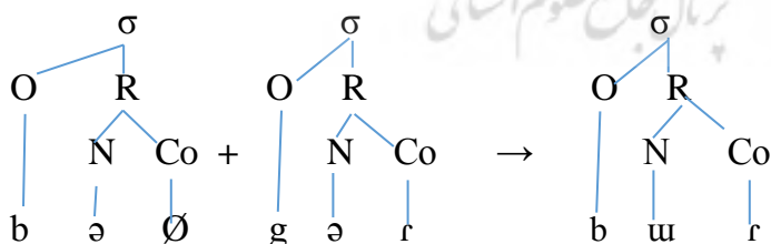
(۸) بازنمایی خودواحد کاهش هجایی واژه [bæʁr] و هجابندی مجدد
