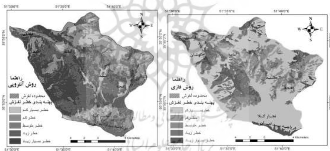
شکل ۶- نقشه‌های طبقه‌بندی شده با استفاده از دو روش ارزیابی فازی و آنتروپی (ترسیم: نگارندگان)
