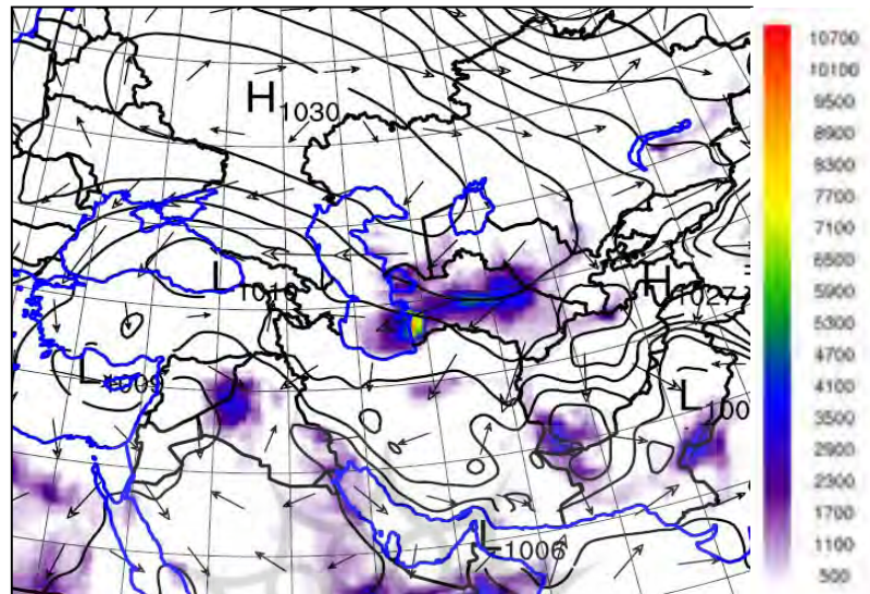
شکل (۹). الگوی فشارسطحی (خطوط هم مقدار بر حسب هکتوپاسکال)، میدان باد ۱۰ متری و غلظت تجمع ریزگردها (پهنه‌های رنگی با واحد میکرو گرم بر مترمکعب) روز ۲۰ سپتامبر ۲۰۱۴ با تفکیک ۳۰ کیلومتر.
