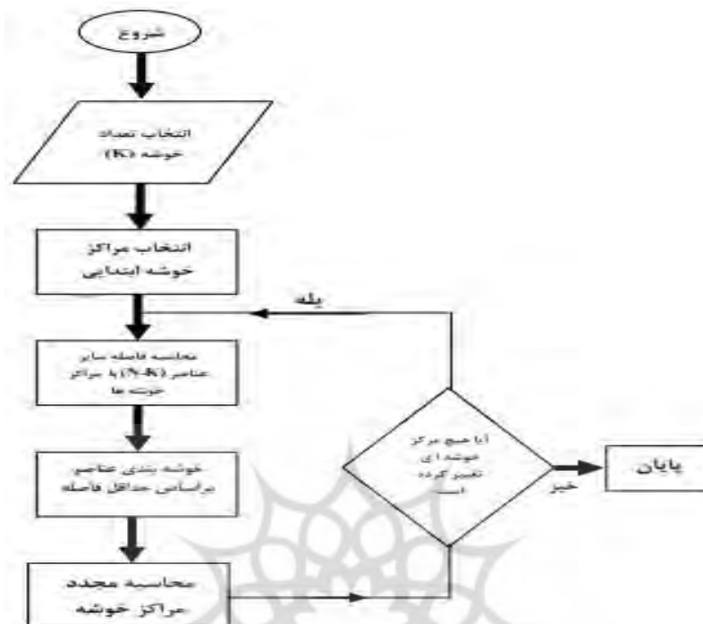
شکل (۱) الگوریتم خوشه‌بندی K-میانگین
