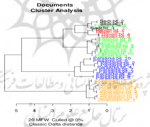
نمودار ۲: تحلیل خوشه‌ای نوشته‌های نویسندگان بر اساس واژه‌های دستوری دو‌نگاشتی در متون ۱۰۰۰۰ واژه‌ای
