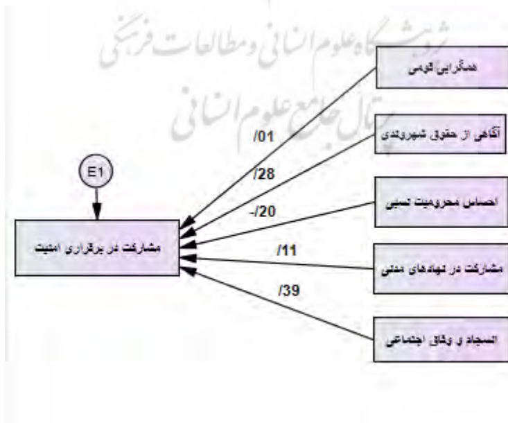
نمودار ۱- نتایج معادله ساختاری متغیرهای پژوهش
