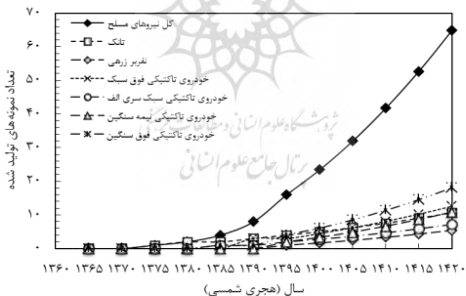
شکل (۳۶) نمودار رشد تعداد نمونه‌های مختلف ادوات و تجهیزات خودرویی تولید شده مرتبط با چشم‌انداز ارتقاء و بروزرسانی سیستم‌های چهارگانه شاسی، موتور، تعلیق و انتقال قدرت خودرو (انباشتی)
