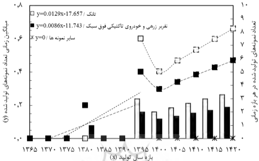
شکل (۲۲) نمودار میانگین زمانی تعداد نمونه‌های مختلف ادوات و تجهیزات خودرویی تولید شده در چشم‌انداز ارتقاء و بروزرسانی سبک‌سازی خودرو و افزایش قابلیت انتقال و جابجایی آن
