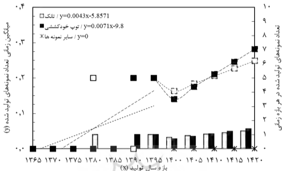
شکل (۲۴) نمودار میانگین زمانی تعداد نمونه‌های مختلف ادوات و تجهیزات خودرویی تولید شده در چشم‌انداز ارتقاء و بروزرسانی شبکه شدن و تبادل داده با سایر ادوات موجود در صحنه نبرد
