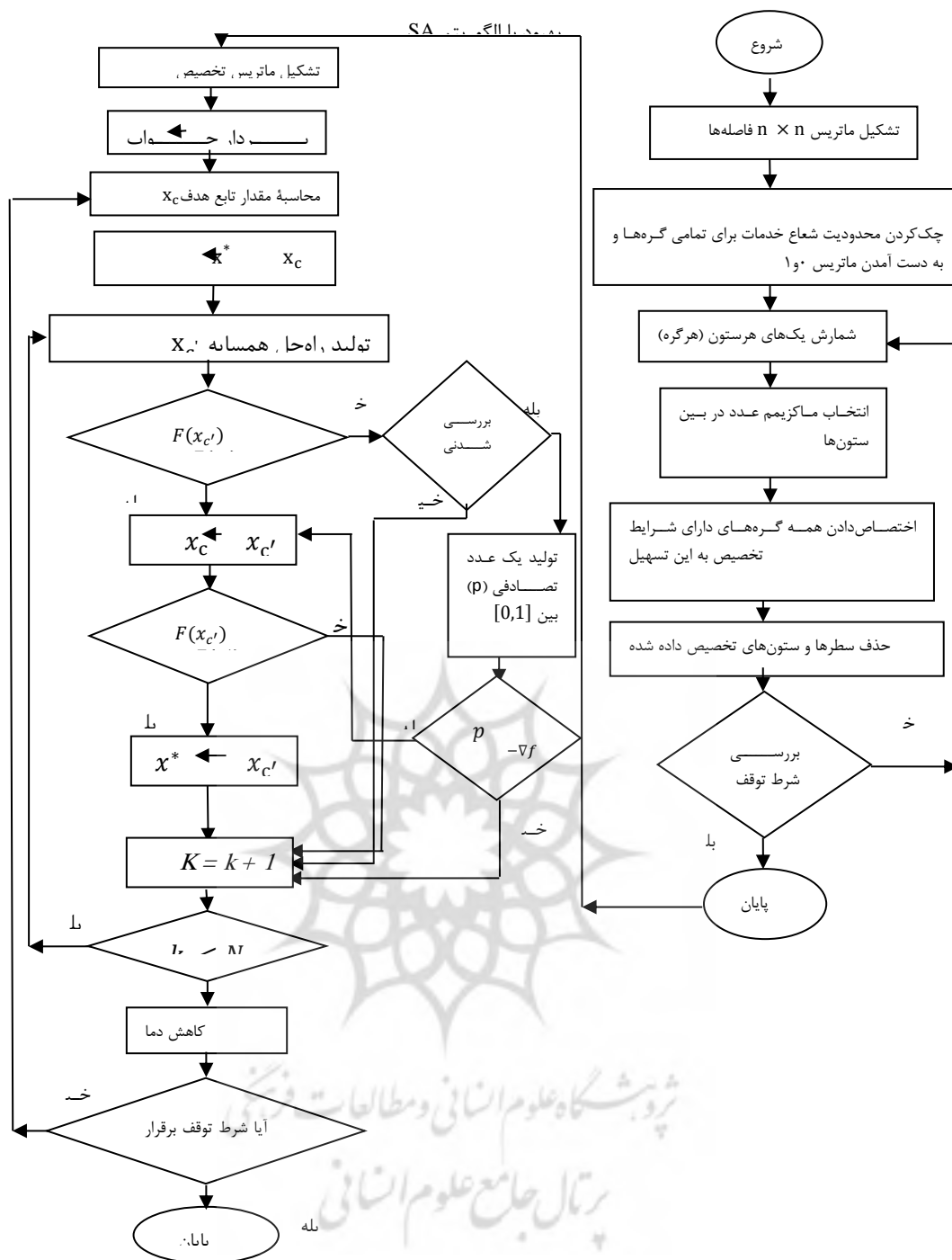
شکل ۷- فلوجارت الگوریتم پیشنهادی
