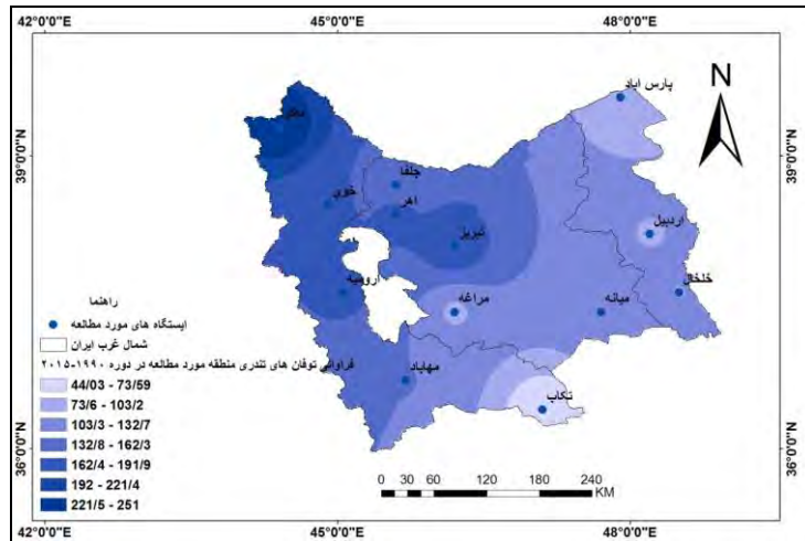
شکل (۶). فراوانی توفان‌های تندری منطقه شمال غرب ایران در دوره آماری (۲۰۱۵-۱۹۹۰)
