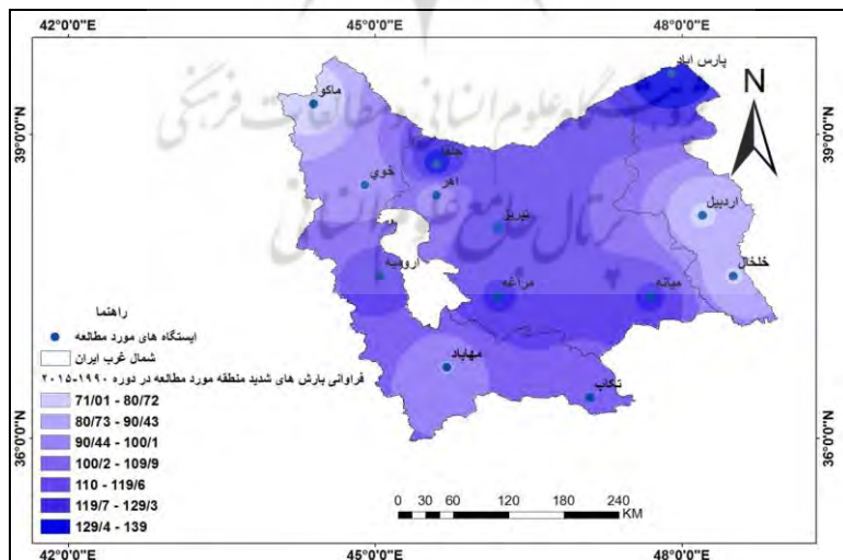
شکل (۷). فراوانی بارش شدید منطقه شمال غرب ایران در دوره آماری (۲۰۱۵-۱۹۹۰)
