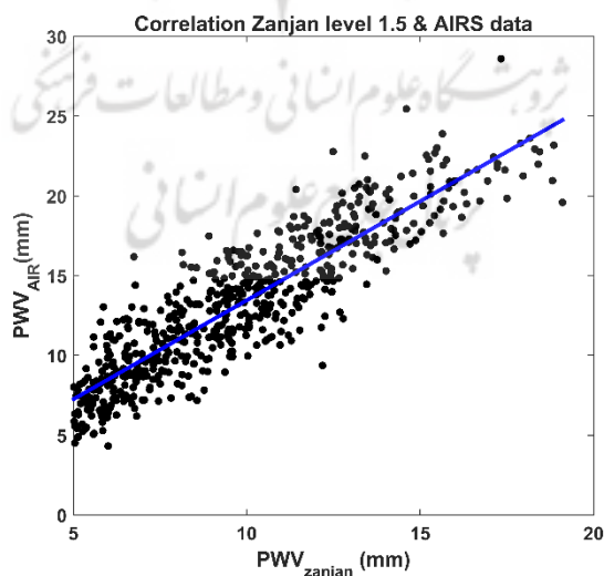
شکل (۳). همبستگی بخار آب قابل بارش (PWV) شیدسنج خورشیدی و سنجنده AIRS در بازه اندازه‌گیری دسامبر
