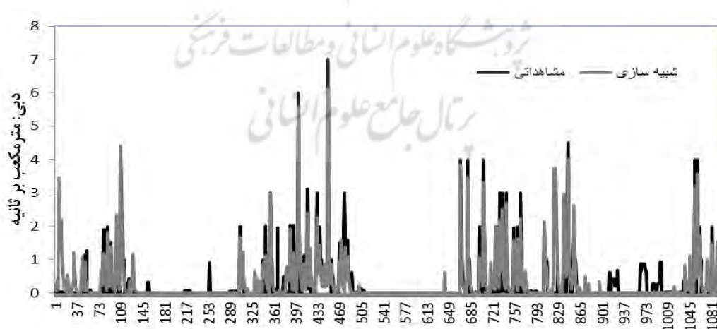
شکل ۶. مقایسه مقادیر دبی مشاهداتی و شبیه‌سازی شده برای دوره واسنجی در حوضه آبخیز گرین
