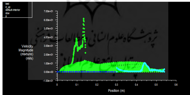
شکل ۷: نحوه تغییر مورفولوژی و سرعت جابجایی توده لغزشی با ویسکوزیته مشخص با استفاده از محاسبه گر fluent
