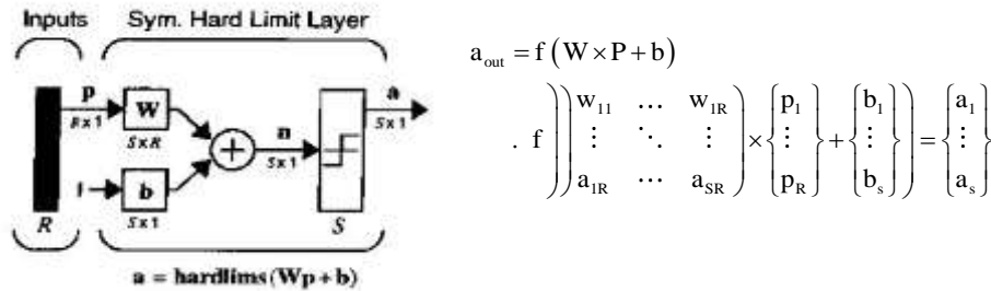
شکل ۲ - شبکه عصبی پرسپترون تک‌لایه (کبا، ۱۳۹۳، ۱۵۸).
