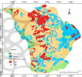
شکل (۴) لایه سنگ‌شناسی منطقه
