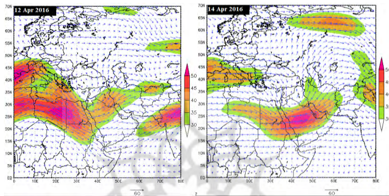
شکل (۶) نقشه رودباد (دامنه رنگ) و بردار باد (بیکان آبی) تراز ۲۵۰ هکتوپاسکال روز ۱۲ و ۱۴ آوریل ۲۰۱۶
