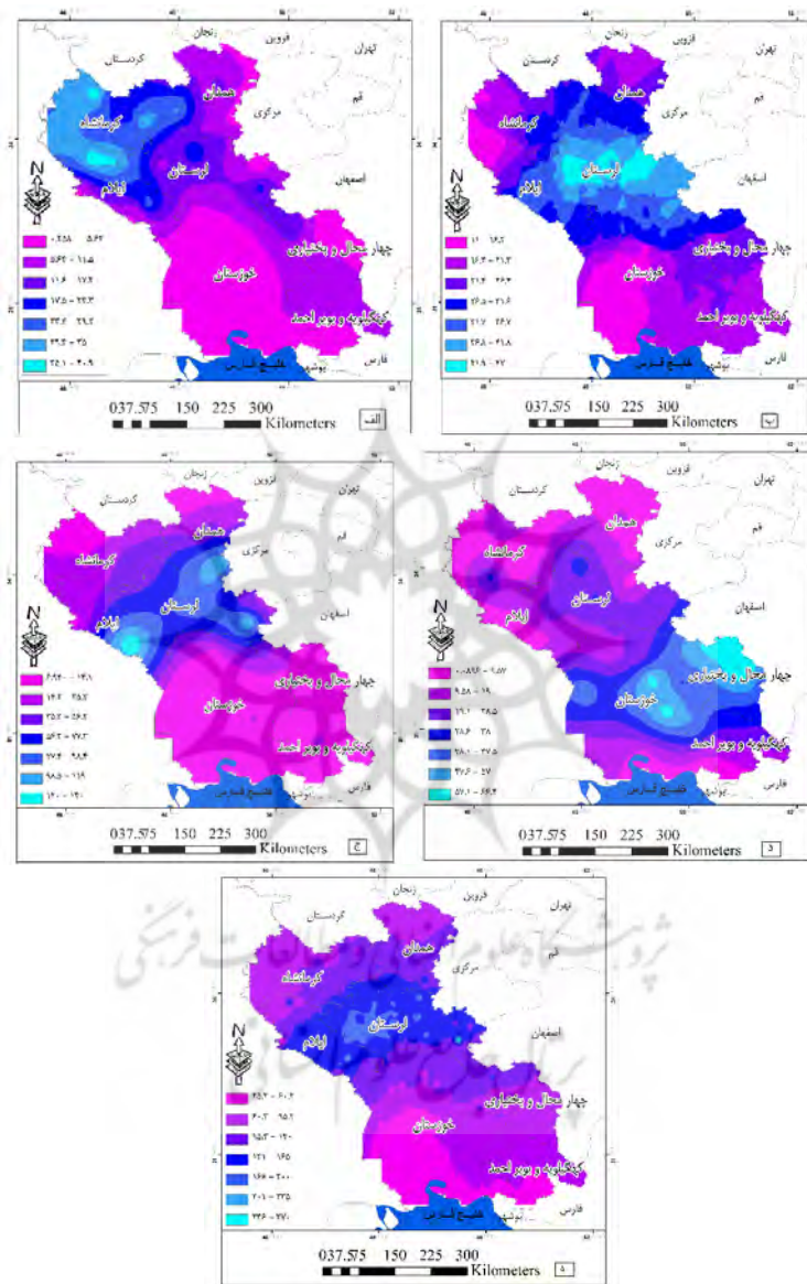
شکل (۲) بیهنه‌بندی بارش روزهای ۱۲ تا ۱۵ آوریل ۲۰۱۶ (به ترتیب الف تا د) و مجموع بارش (ه)
