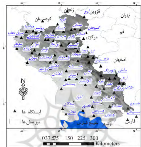
شکل (۱) محدوده جغرافیایی منطقه پژوهش و ایستگاه‌های هواشناسی مورد استفاده
