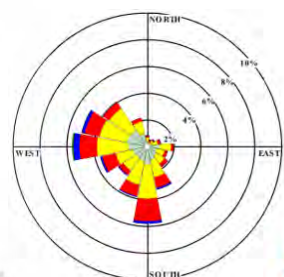
شکل ۱. سرعت و جهت باد در ایستگاه اردل
