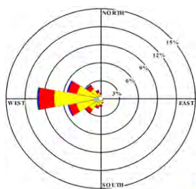
شکل ۳. سرعت و جهت باد در ایستگاه کوهرنگ
