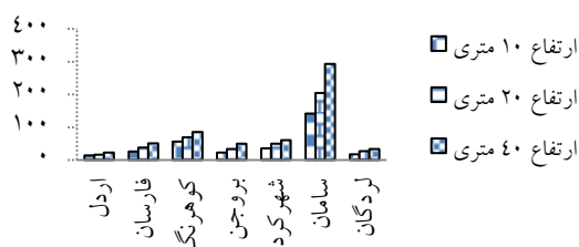
شکل ۹. چگالی توان بادی سالیانه به تفکیک
