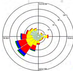
شکل ۵. سرعت و جهت باد در ایستگاه شهرکرد
