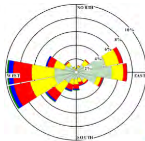
شکل ۴. سرعت و جهت باد در ایستگاه بروجن
