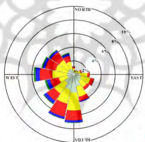
شکل ۲. سرعت و جهت باد در ایستگاه فارسان
