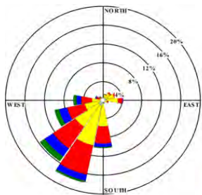
شکل ۶. سرعت و جهت باد در ایستگاه سامان
