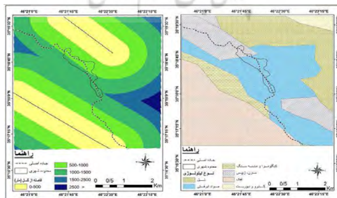
شکل ۵- پارامترهای زمین‌شناسی
