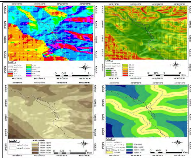
شکل ۴- پارامترهای ژئومورفولوژیکی
