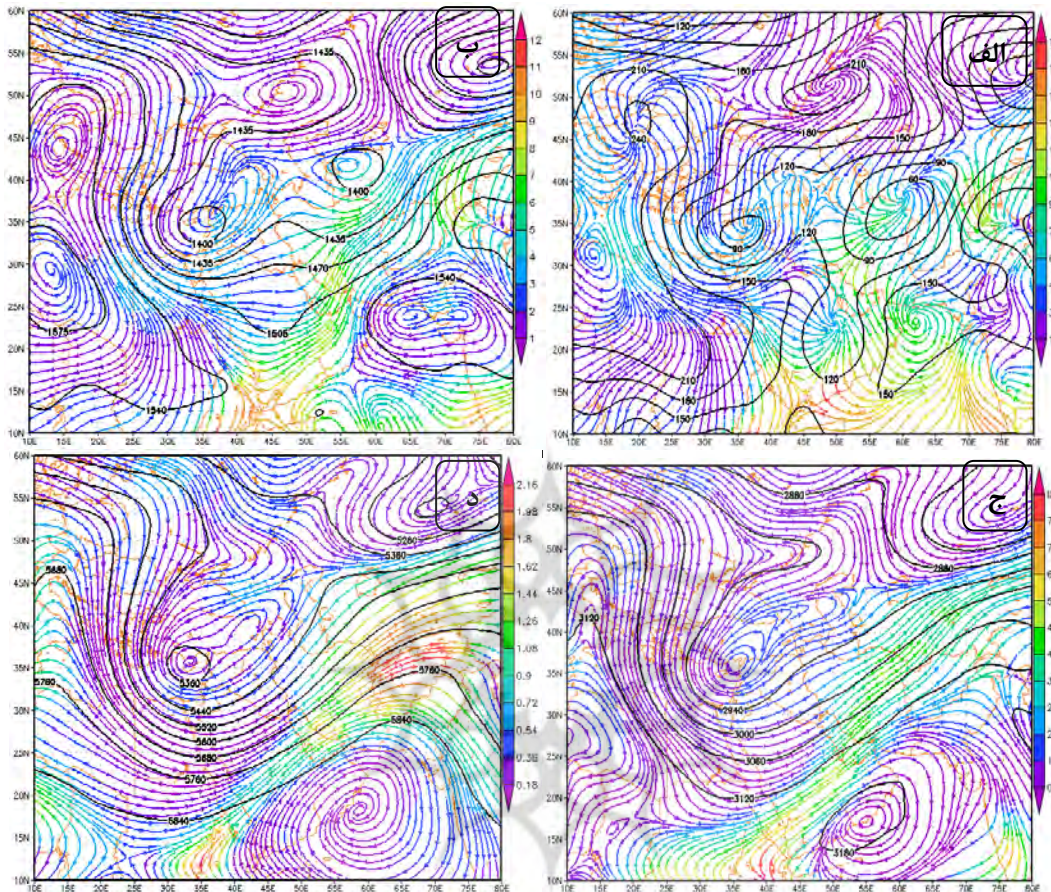
شکل ۹). نقشه‌های ترکیبی وزش رطوبتی و ارتفاع ژئوپتانسیل در ترازهای الف: ۱۰۰۰، ب: ۸۵۰، ج: ۷۰۰، د: ۵۰۰ هکتوپاسکال در روز ۲۵ فوریه ۱۹۹۲
