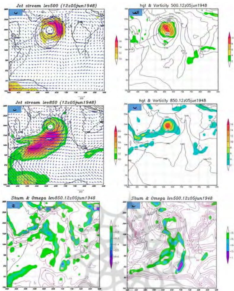
شکل ۲- الف تا ج به ترتیب: ارتفاع ژئوپتانسیل و فرارفت تاوایی تراز ۵۰۰ میلی بار، رودباد تراز ۵۰۰ میلی بار، ارتفاع ژئوپتانسیل و فرارفت تاوایی تراز ۸۵۰ میلی بار، رودباد تراز ۸۵۰ میلی بار، نم و ویژه و سرعت قائم تراز ۵۰۰ و ۸۵۰ میلی بار
