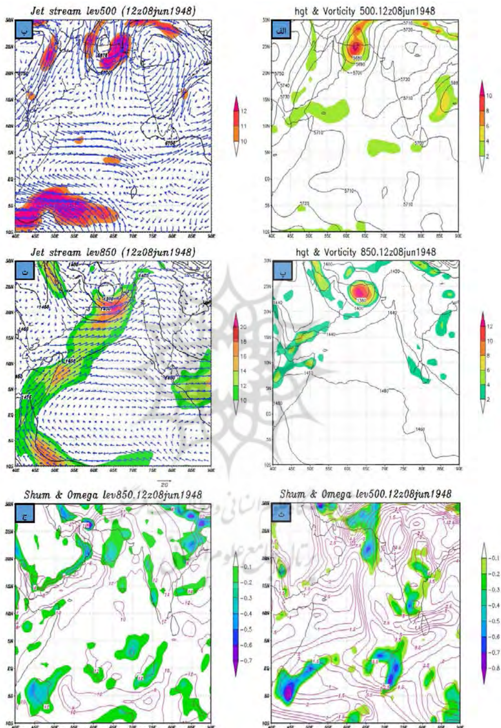
شکل ۶- الف تا ج به ترتیب ارتفاع ژئوپتانسیل و فرافرت تاوایی تراز ۵۰۰ میلی بار، رودباد تراز ۵۰۰ میلی بار، ارتفاع ژئوپتانسیل و فرافرت تاوایی تراز ۸۵۰ میلی بار، رودباد تراز ۸۵۰ میلی بار، نم ویژه و سرعت قائم تراز ۵۰۰ میلی بار و نم ویژه و سرعت قائم
