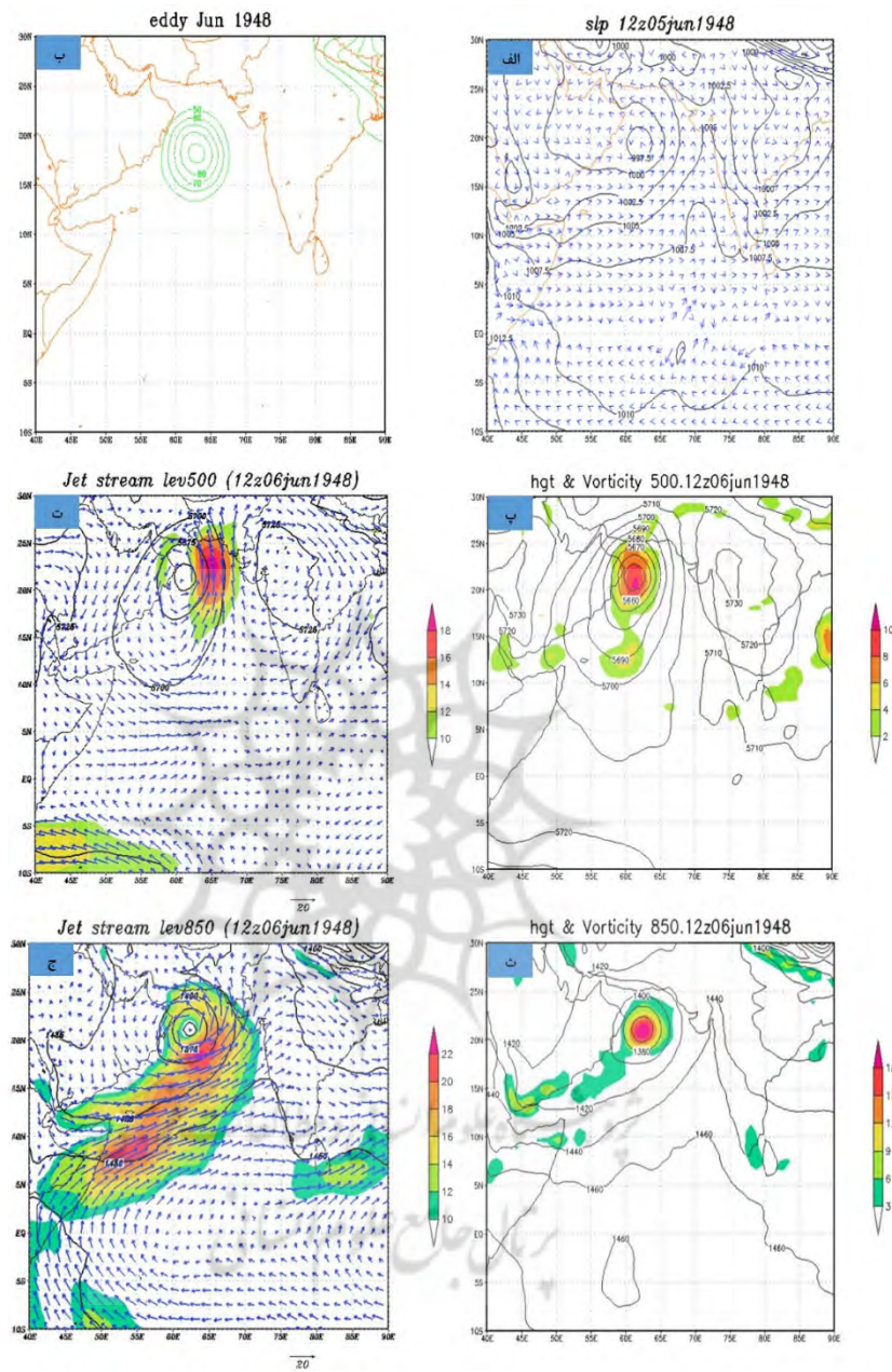
شکل ۳- الف تا ج به ترتیب فشار تراز دریا، بیجانہ جوی تراز ۵۰۰ میلی بار (ساعت ۱۲ روز ۰۵ ژوئن ۱۹۴۸)، ارتفاع ژئوپتانسیل و فرارفت تاوایی تراز ۵۰۰ میلی بار، رودباد تراز ۵۰۰ میلی بار، ارتفاع ژئوپتانسیل و فرارفت تاوایی تراز ۸۵۰ میلی بار و رودباد تراز ۸۵۰ میلی بار ساعت ۱۲ روز ۰۶ ژوئن ۱۹۴۸
