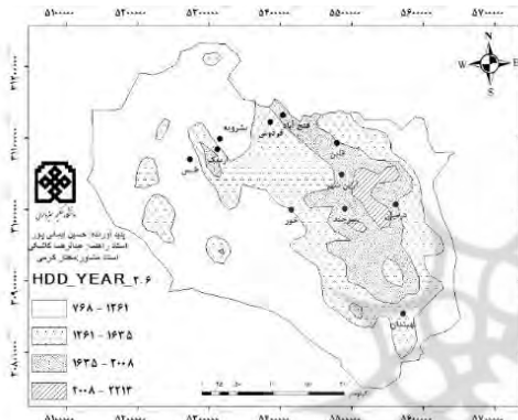
شکل (۳۱). پراکنش مکانی نیازهای گرمایشی سالانه دوره آینده (۲۰۱۶-۴۱)، سناریو RCP_2.6
