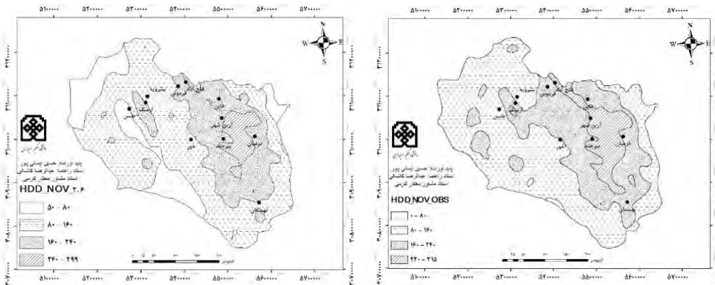
شکل (۱۰). پراکنش مکانی نیازهای گرمایشی ماه آبان در دوره مشاهده ای (۱۹۹۰-۲۰۱۵) شکل (۱۱). پراکنش مکانی نیازهای گرمایشی آبان در دوره
