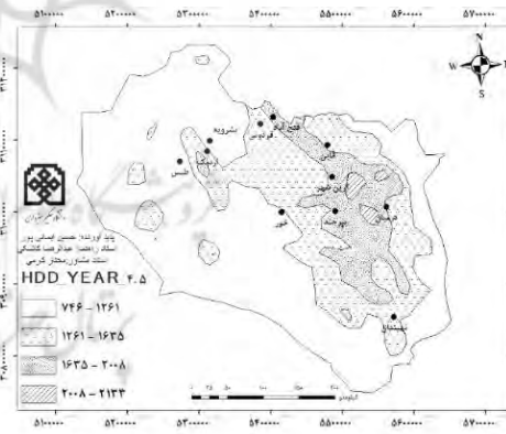
شکل (۳۲). پراکنش مکانی نیازهای گرمایشی سالانه دوره آینده (۲۰۱۶-۴۱) سناریو RCP_4.5
