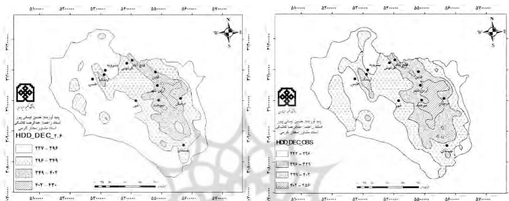
شکل (۱۴). پراکنش مکانی نیازهای گرمایشی آذر در دوره مشاهده ای (۱۹۹۰-۲۰۱۵) و شکل (۱۵). پراکنش مکانی نیازهای گرمایشی آذر در دوره آینده (۲۰۱۶-۴۱) سناریو RCP_2.6
