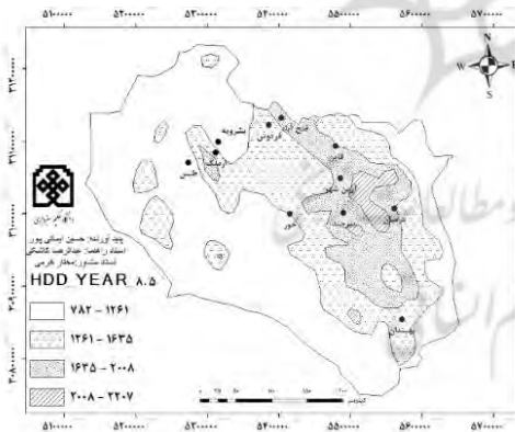
شکل (۳۳). پراکنش مکانی نیازهای گرمایشی سالانه دوره آینده (۲۰۱۶-۴۱)، سناریو RCP_8.5
