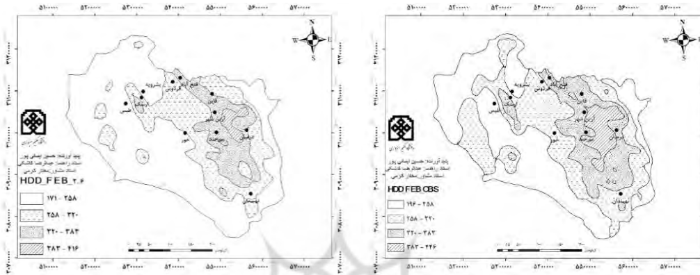
شکل (۲۲). پراکنش مکانی نیازهای گرمایشی ماه بهمن در دوره مشاهده ای (۱۹۹۰-۲۰۱۵) و پراکنش مکانی نیازهای گرمایشی ماه بهمن در دوره آینده (۲۰۱۶-۴۱)، سناریو RCP_2.6
