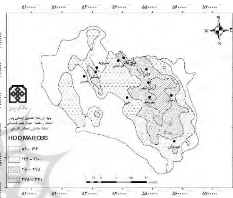
شکل (۲۶). پراکنش مکانی نیازهای گرمایشی ماه اسفند در دوره مشاهده‌ای (۱۹۹۰-۲۰۱۵)
