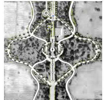
تصویر ۶: بزرگ‌نمایی عناصر بخش مرکزی باغ، محور خیابان از محل شروع انشعابات جانبی، ردیف حوض‌ها و جوی آب. تفکیک مسیر پیاده (خاکستری) و سواره (سفید) در نقشه مشخص شده است.
