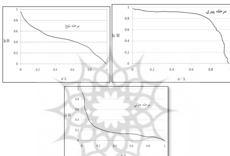
شکل ۴: منحنی های هیپسومتری نظری چرخه فرسایش کلر و همکاران، ۲۰۰۲
