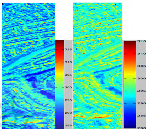
نگاره ۵: به ترتیب از راست به چپ الف) تصویر دمایی محصول سنجنده های تس ب) تصویر دمایی بدست آمده از الگوریتم ARTEMISS
