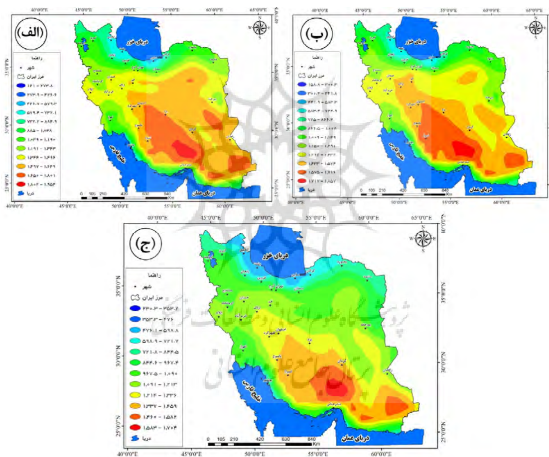
شکل ۵: ارتفاع لایه مرزی (BLH) بر فراز ایران در فصل تابستان، (الف) ژوئای، (ب) آگوست، (ج) سپتامبر
