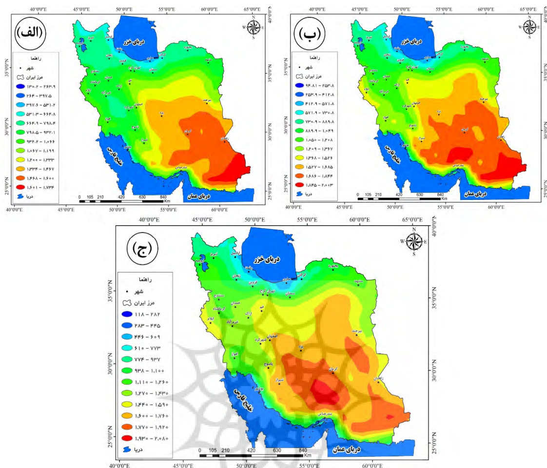
شکل ۴: ارتفاع لایه مرزی (BLH) بر فراز ایران در فصل بهار، الف) آوریل، ب) می، ج) ژوئن
