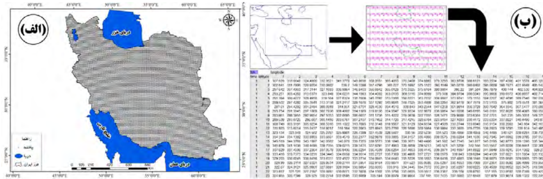
شکل ۱: (الف) یاخته‌های ۰/۱۲۵×۰/۱۲۵ درجه قوسی مرکز پیش‌بینی میان‌مدت هواسپهر اروپایی (ECMWF)
