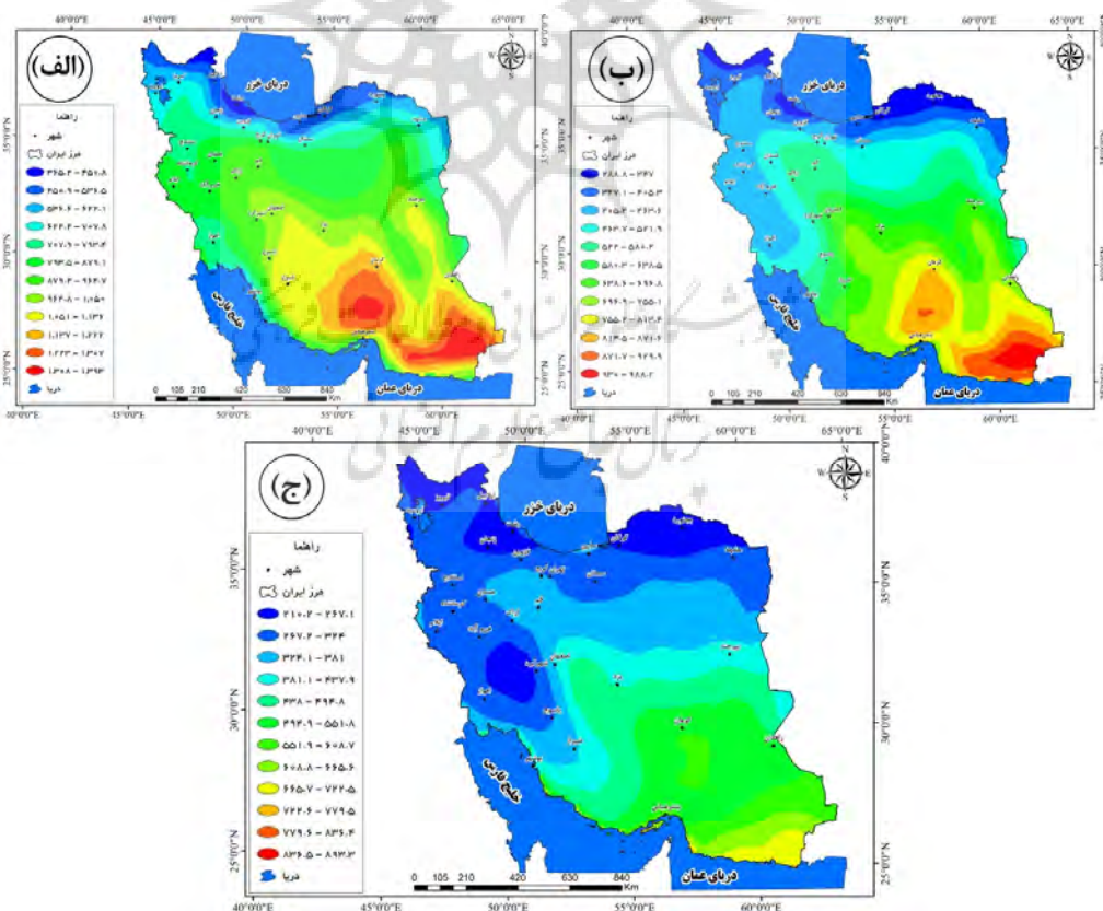
شکل ۶: ارتفاع لایه مرزی (BLH) بر فراز ایران در فصل پاییز، (الف) اکتبر، (ب) نوامبر، (ج) دسامبر
