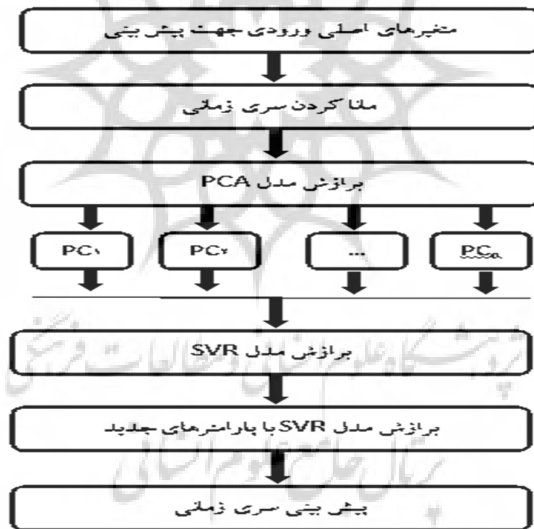
شکل (2): الگوریتم کلی مدل پیش‌بینی
