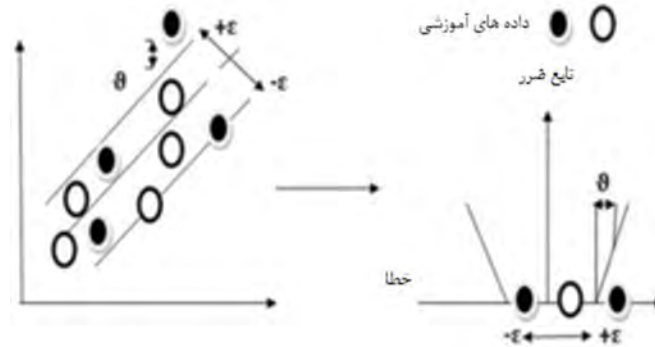
شکل (1): تابع ضرر و پینک و متغیرهای slack
