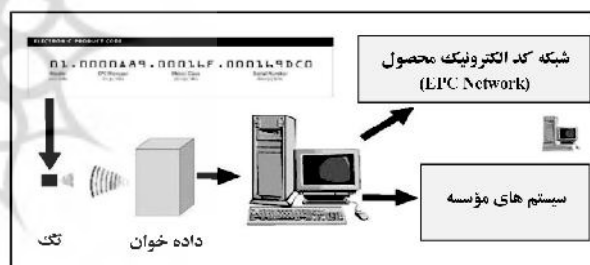
نمودار ۱- اجزای سیستم RFID
