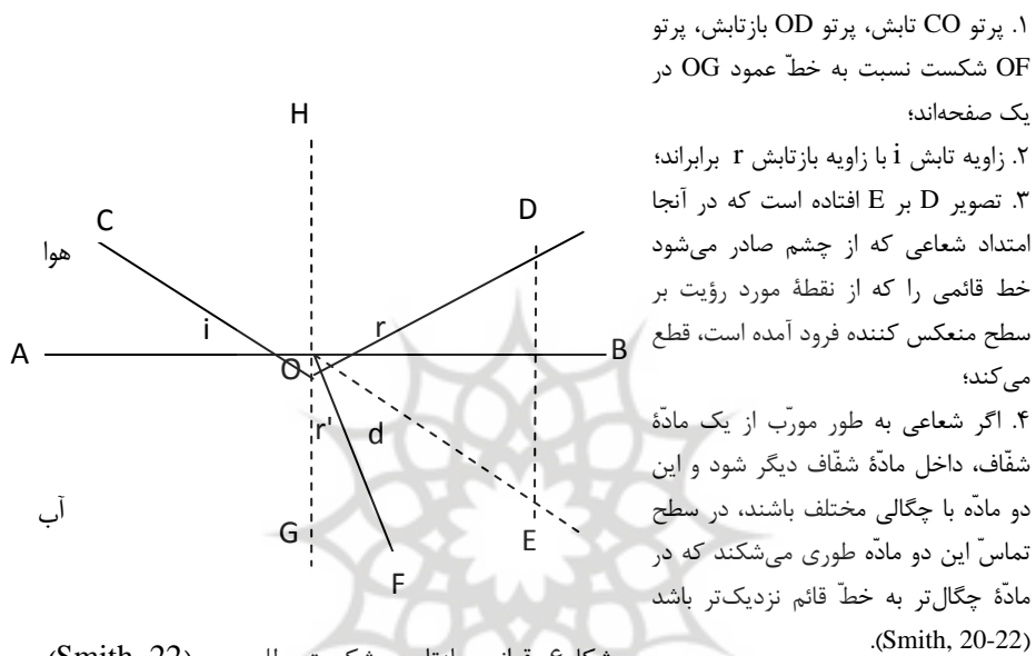
شکل ۶- قوانین بازتاب و شکست بطلمیوس (Smith, 22).
