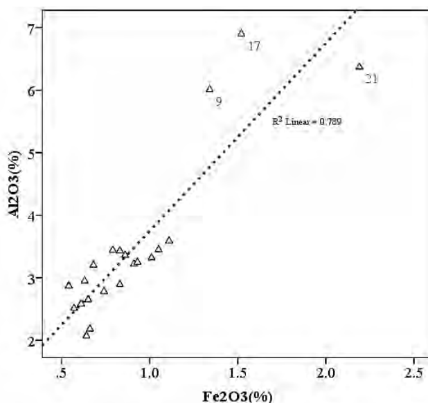
شکل ۴: تغییرات درصد وزنی اکسید آهن برحسب اکسید آلومینیم (آلمینا) در نمونه‌های آنالیز شده محوطه شاتور
