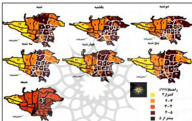
شکل (۱۲): مناطق مختلف شهر تهران بر اساس غلظت منوکسیدکربن برحسب نوع روز
