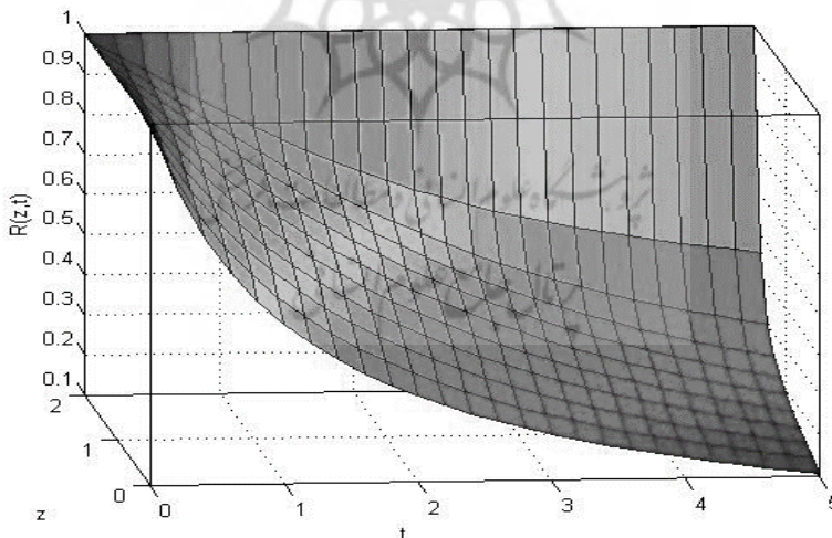
شکل ۱: جواب عددی مثال ۲ با مؤلفه‌های \alpha_1 = \alpha_2 = 1
