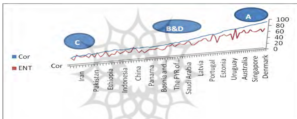
نمودار ۶. توزیع کشورها براساس میانگین رتبه ۵ ساله فساد و کارآفرینی
