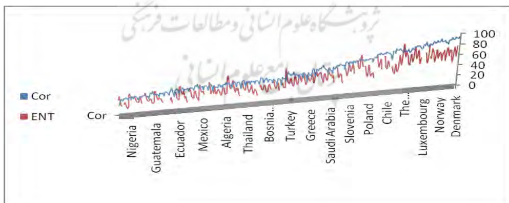
نمودار ۷. توزیع کشورها براساس رتبه سالانه فساد و کارآفرینی
