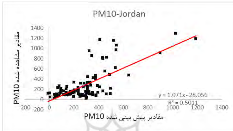
شکل (۹). نمودار پراکنش خروجی مدل Jordan با داده‌های واقعی
