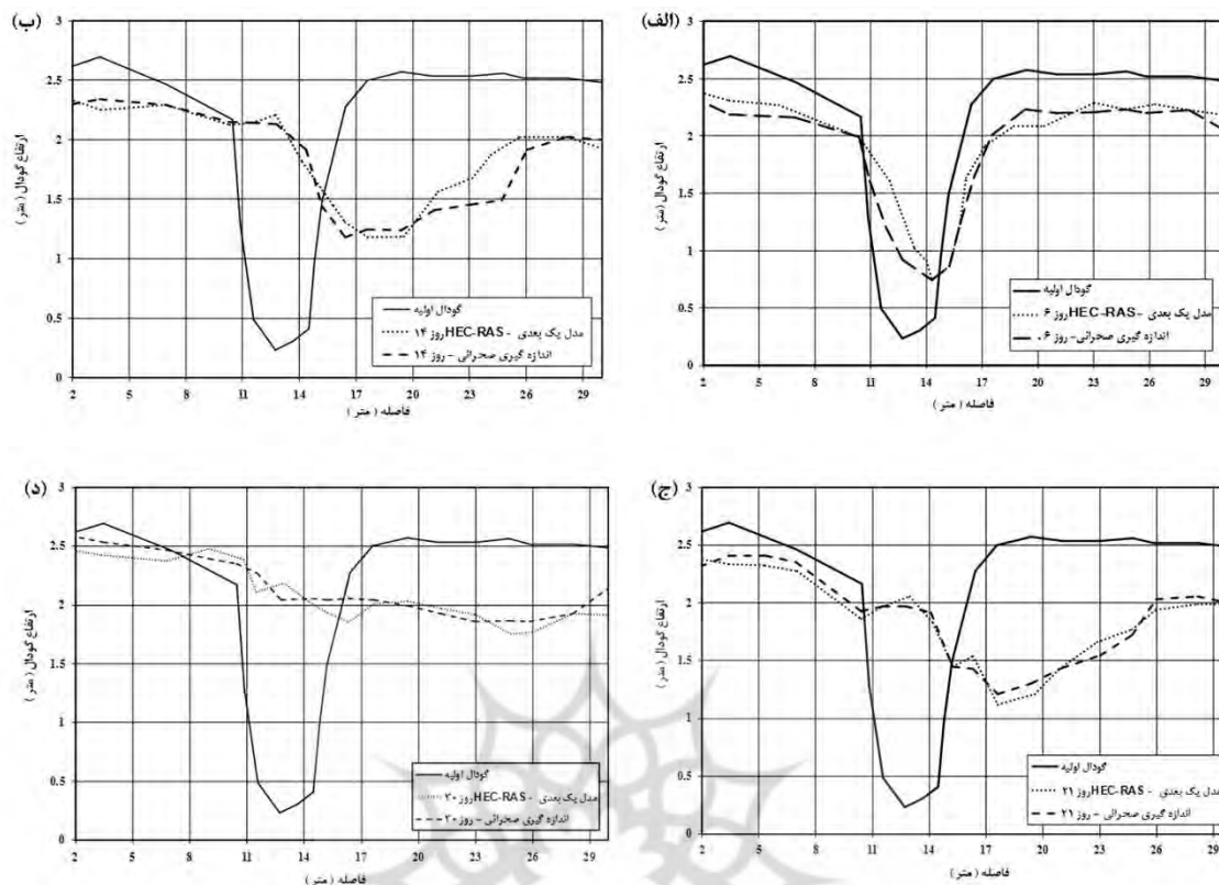
شکل ۵: مقایسه بین نتایج حاصل از شبیه سازی عددی مدل یک بعدی و اندازه گیری‌های صحرانی حرکت گودال: (الف) روز ۶، (ب) روز ۱۴، (ج) روز ۲۱، (د) روز ۳۰
