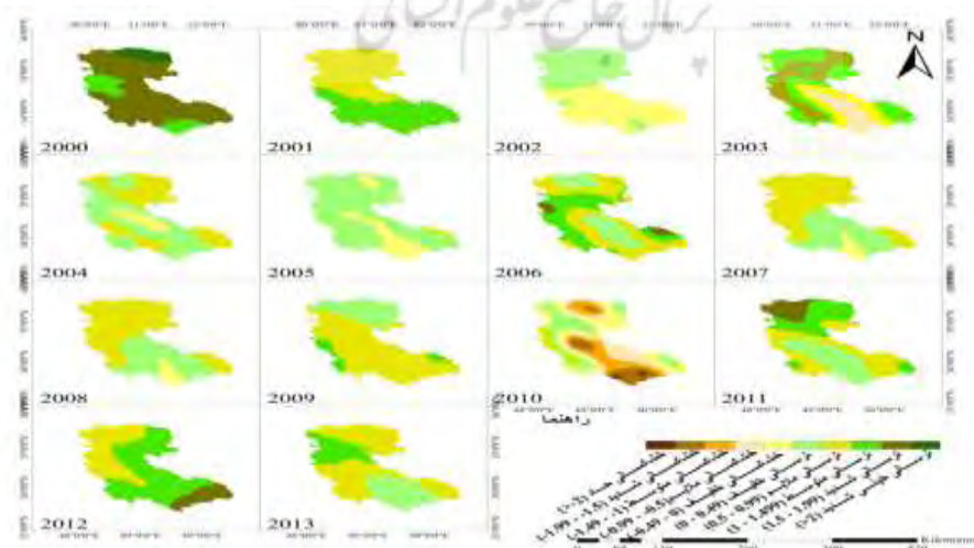
شکل ۵: پهنه بندی خشکسالی استان مرکزی با استفاده از شاخص بارش استاندارد (SPI) فصلی (۲۰۰۰-۲۰۱۳)
