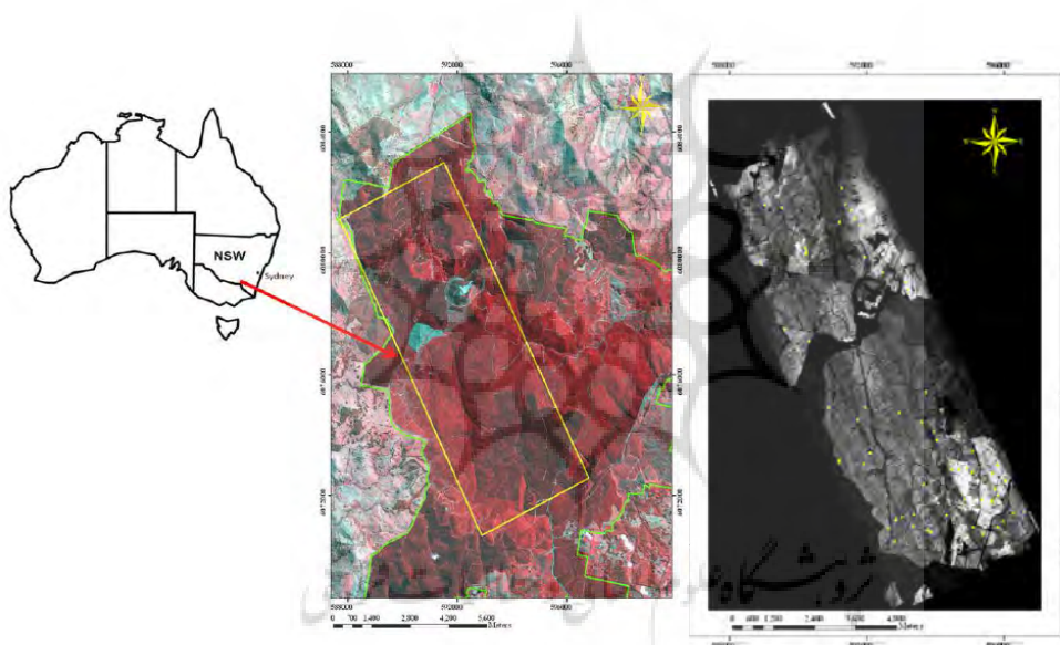
شکل ۱. الف- کادر زرد نشان‌دهنده منطقه مورد مطالعه در این تحقیق بر تصویر رنگی کاذب ۳ ماهواره اسپات-۵؛ ب- لایه CHM به‌دست‌آمده از داده‌های لیدار، نقاط زرد رنگ بر این لایه معرف موقعیت مکانی پلات‌های برداشت شده
