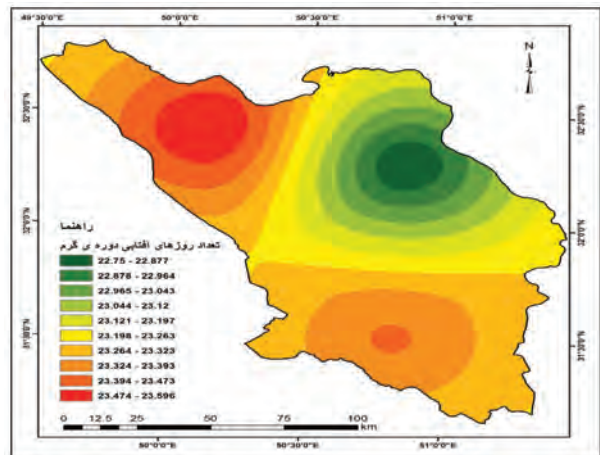
نگاره ۸: تعداد روزهای آفتابی دوره گرم در استان چهارمحال و بختیاری
