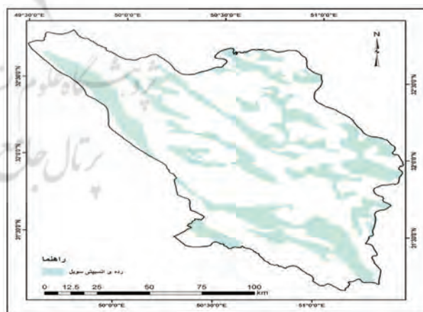
نگاره ۵: مناطق دارای خاک رده اینسیپتی سویل در سطح استان چهارمحال و بختیاری
