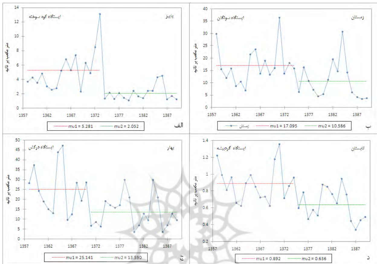
نگاره ۲: تغییرات دبی در ایستگاه‌های کوه سوخته، سولگان، درکش و گردپیشه در دوره آماری ۱۳۵۸ تا ۱۳۸۹ (خط‌های نقطه چین میانگین سری‌های قبل و بعد از نقطه تغییر می‌باشند)
