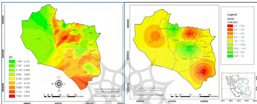
شکل ۱۰: توزیع EC منابع آب استان مأخذ: نگارندگان، ۱۳۹۶
